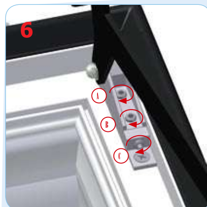
Regulace polohy křídla v rámu (pouze servis). A, B - přitlačné šrouby C - regulační šroub
