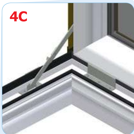
Zajištěná otevírací / zavírací zarážka - zajištěná poloha, otevřené křídlo 90°
